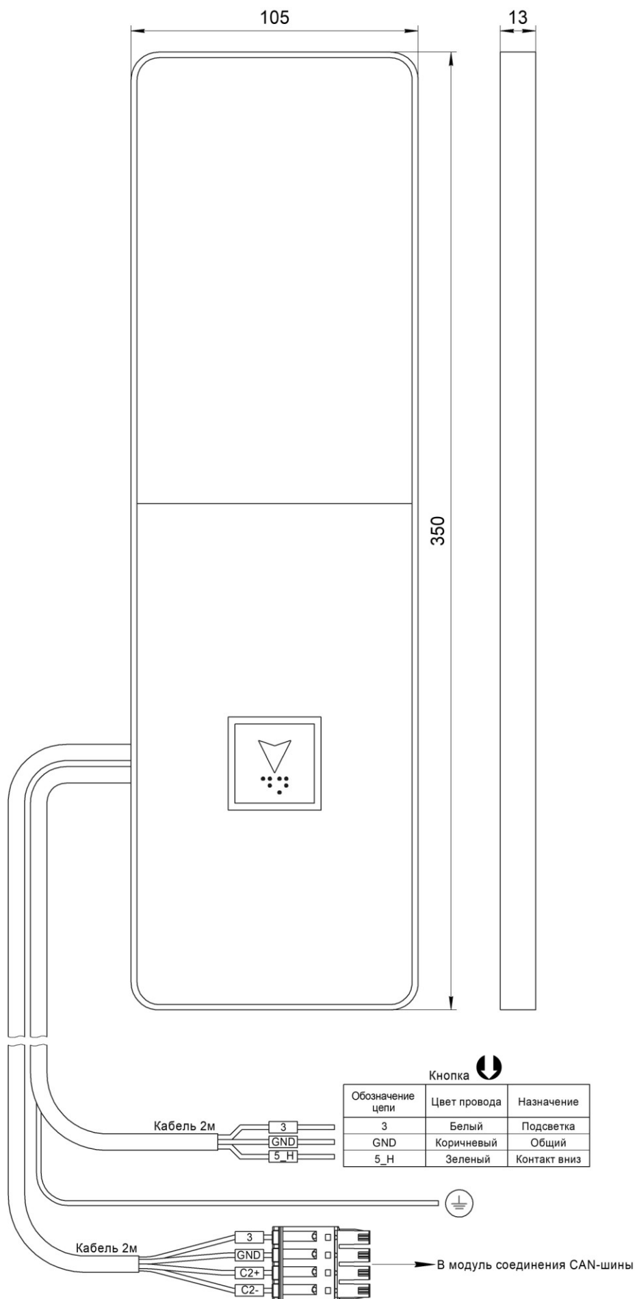
Рис.1 Внешний вид, габаритные и установочные размеры Вызывного поста МАЛАХИТ НШЕК.468381.086
